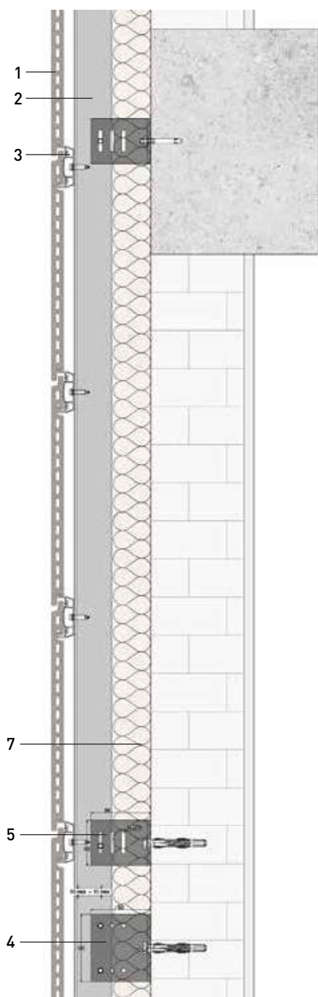
A Vertical section Sección vertical
