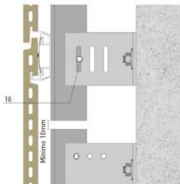
C Fixation between vertical profiles Fijación entre perfiles verticales
