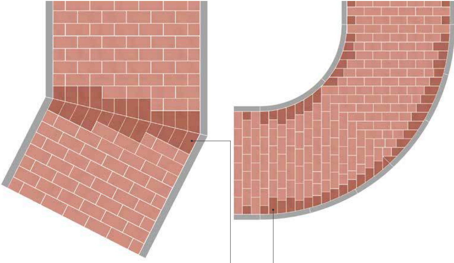
Abb. A5-12: Gehung mit Zuschnitt der Passsteine zugearbeitete Pflasterklinker
