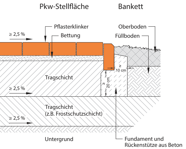
Abb. 5-13: Randeinfassung durch Tiefbordsteine
